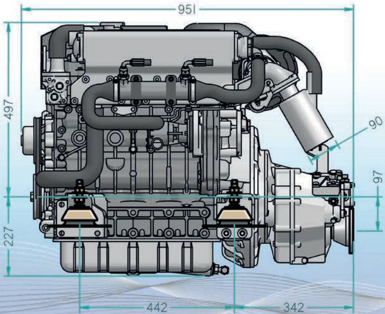
Dimensions typiques: visitez notre site web pour obtenir tous les dessins ou bien contactez Beta Marine
