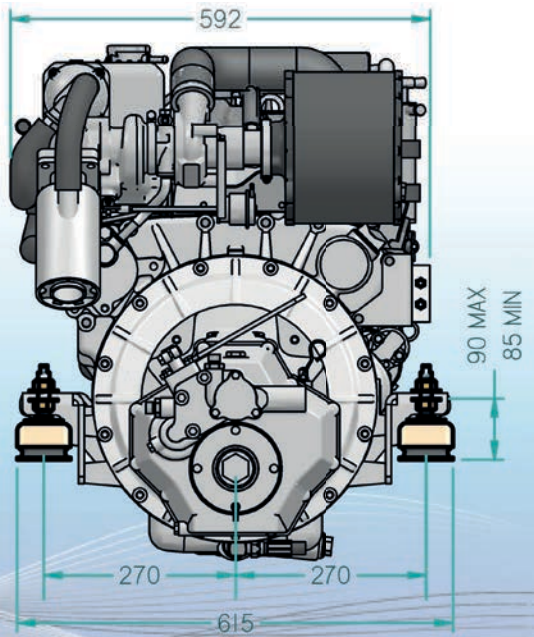
Dimensions typiques: visitez notre site web pour obtenir tous les dessins ou bien contactez Beta Marine
